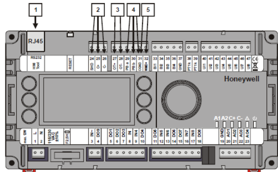
图4. 总线及端口连接
