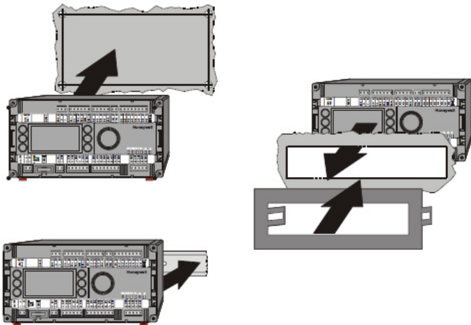
图3. 安装方式
