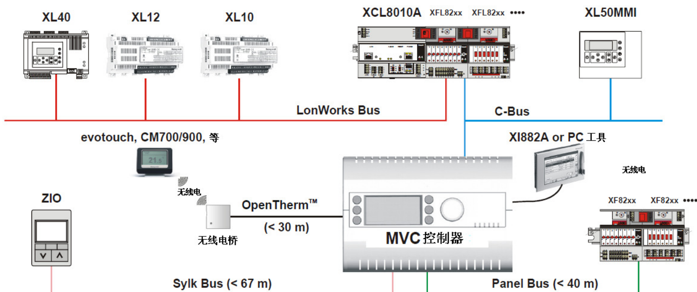
图1. MVC 控制器与Excel 5000系统结构
