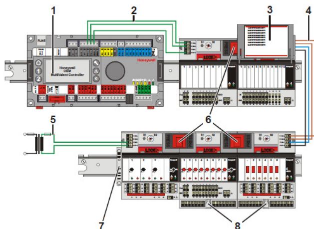
图 7. 安装与DIN导轨上的MVC 控制器及 Panel Bus I/O 模块
