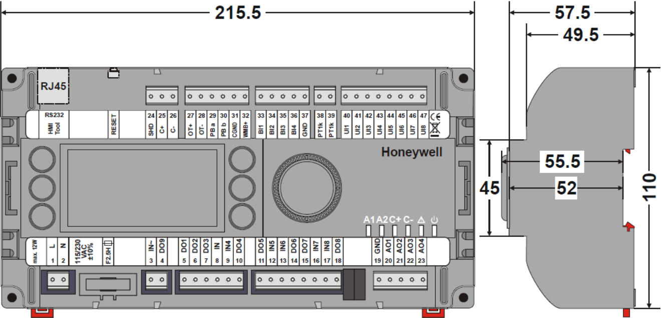
图9. MVC 控制器 (MVC-80M-CPSW1A, 无端子盖和端子), 外形尺寸 (mm)
